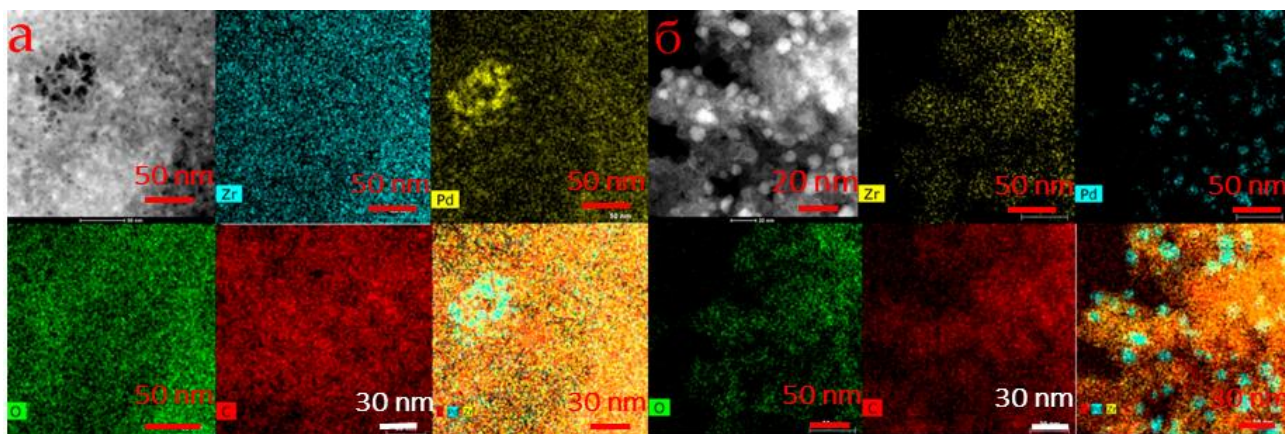
Рисунок 11 – Картирование поверхности катализатора по элементам (O, C, Zr и Pd) а) \text{Pd/Zr}_6\text{O}_4(\text{OH})_4(\text{ТФК-NH}_2)_6 ; б) \text{Pd/Zr}_6\text{O}_4(\text{OH})_4(\text{ТФК})_6
