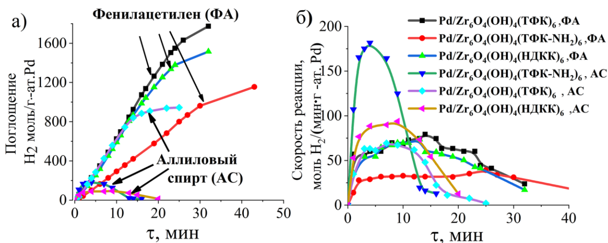
Рисунок 13 – а) Зависимости расхода водорода от времени в повторных циклах при гидрировании фенилацетилена и аллилового спирта; б) Скорость расходования H 2 в повторных циклах (масса навески катализатора – 0.05 г, температура 40°C, давление H 2 – 0.1 МПа, растворитель – этанол, объем субстрата – 0.25 мл).
