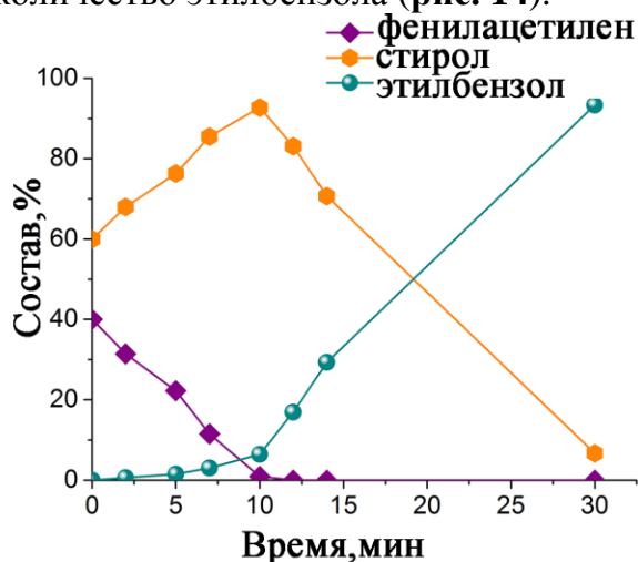
Рисунок 14 – Зависимость состава реакционной смеси от времени при гидрировании смеси ФА и стирола при мольном соотношении стирол: ФА = 3:2 (масса навески Pd/Zr_6O_4(OH)_4(НДКК)_6 – 0.05 г, температура 40°C, давление H 2 – 0.1 МПа, растворитель – этанол, объем субстрата – 0.25 мл).
