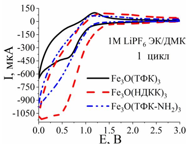
Рисунок 8 – ЦВА ячеек \text{Li}/\text{МОКП} с 1\text{M LiPF}_6 в смеси ЭК/ДМК (1:1) в диапазоне 0.01–3.0, скорость 1мВ/с
