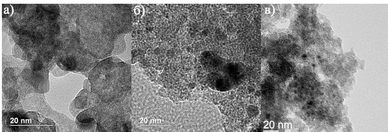
Рисунок 12 – ПЭМ–изображение поверхности катализаторов \text{Pd/Zr}_6\text{O}_4(\text{OH})_4(\text{ТФК})_6 (а), \text{Pd/Zr}_6\text{O}_4(\text{OH})_4(\text{ТФК-NH}_2)_6 (б) и \text{Pd/Zr}_6\text{O}_4(\text{OH})_4(\text{НДКК})_6 (в)
