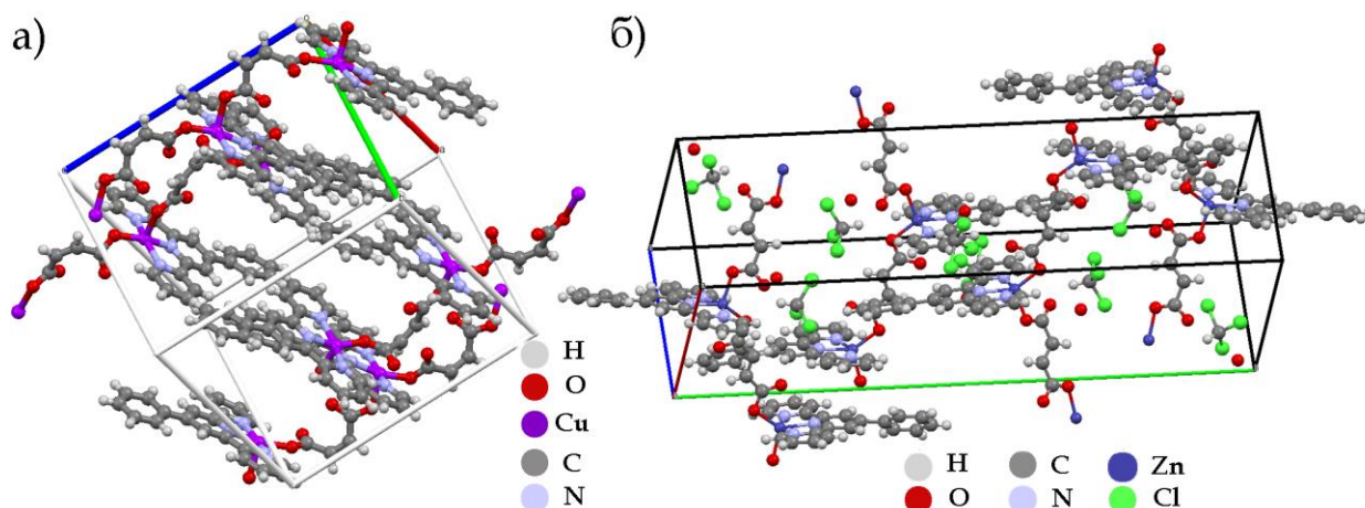
Рисунок 2 – Элементарная ячейка координационного полимера CuMaleatePhtpy (а) и ZnMaleatePhtpy (б)
