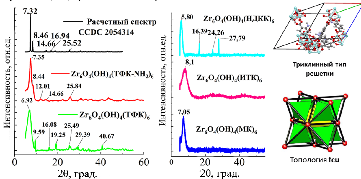
Рисунок 9 – Рентгеновские дифрактограммы полученных МОКП
